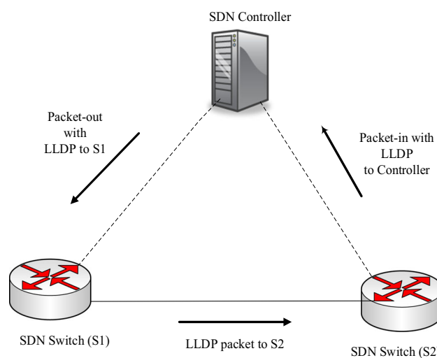
Fig. 3 LLDP in SDN
